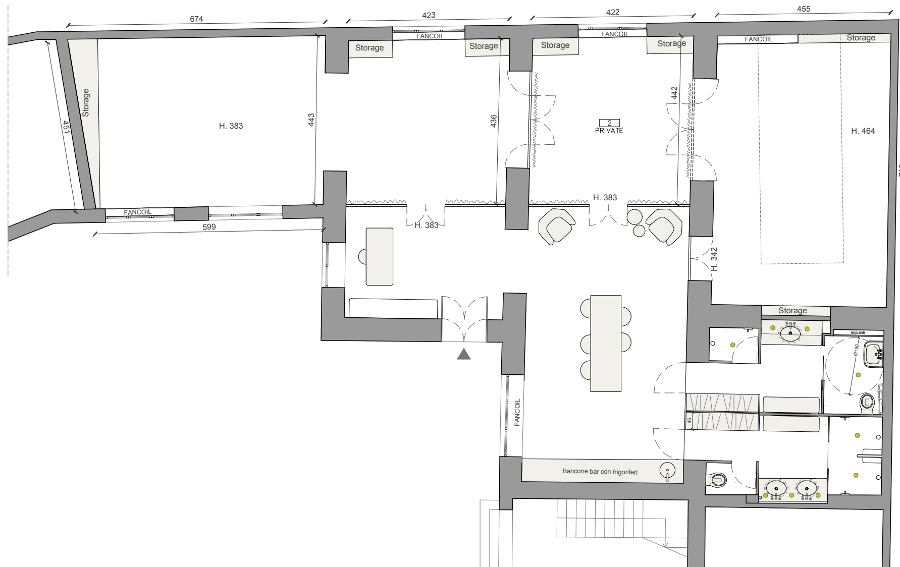
01 PIANTA 1:100
