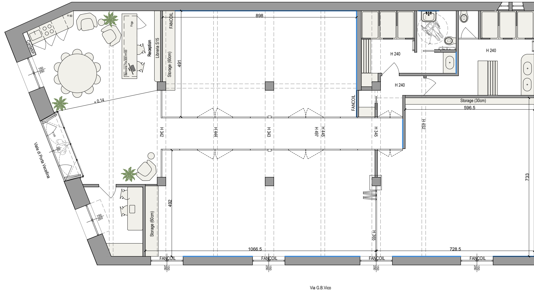
01 PIANTA 1:100
